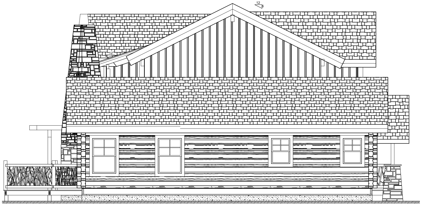
RIGHT ELEVATION
